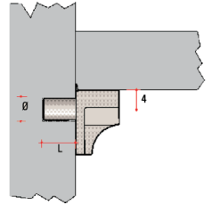
Artikel: 3170900 vernikkeld / transparant Ø=5mm / L=8mm SD13
