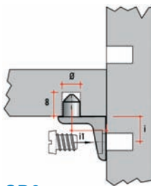
Artikel: kunststof wit kunststof bruin kunststof zwart Ø=12mm / L=9mm / L1-10,5mm
