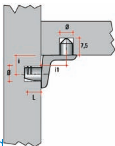
Artikel: 3170915 vernikkeld 3170916 messing 3170917 gebronsd Ø=5mm / L=16mm GD2
